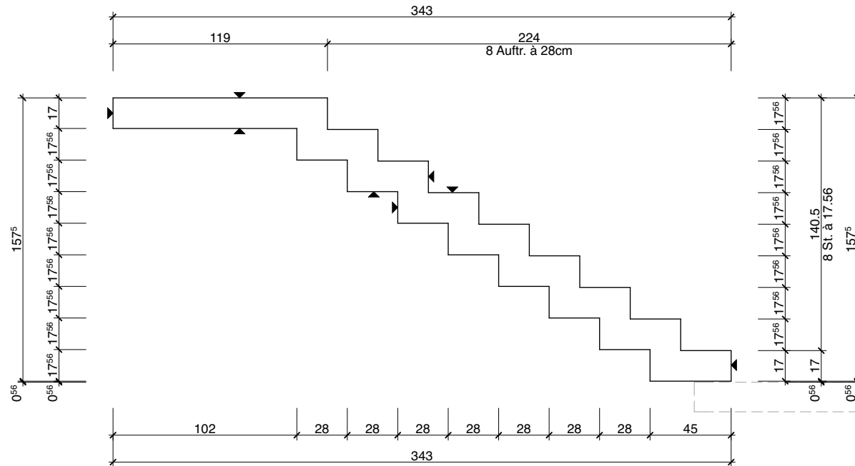
Ansicht seitlich
