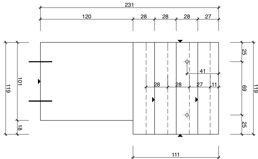
Aufsicht
