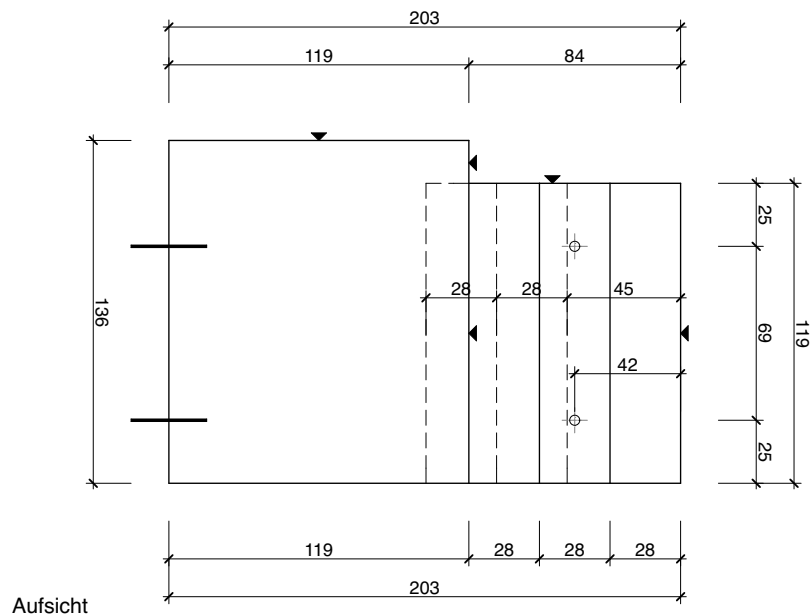
Aufsicht
